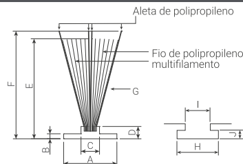
QUADRA-FIN (QF)
