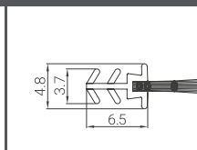
PROFILE: KP (Kerf pile)
