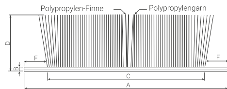
DUST-PLUG (DP)
