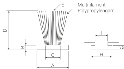
POLY-BOND (PB)
