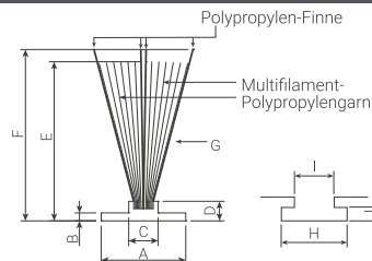
QUADRA-FIN (QF)
