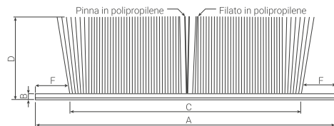
DUST-PLUG (DP)
