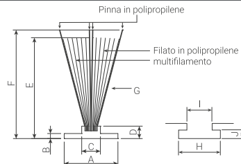
QUADRA-FIN (QF)
