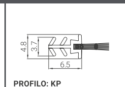
PROFILO: KP (spazzolino per cava)
