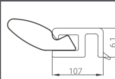
PERFIL: 2165626
