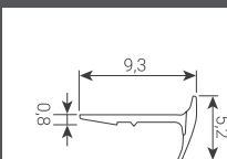
PERFIL: 1034
