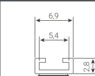
PERFIL: 5594
