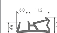
PERFIL: 1034
