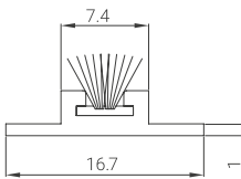
PERFIL: 5060
