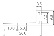
PERFIL: 3016
