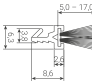
PERFIL: 908
