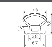
PERFIL: 1509
