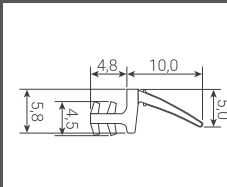
PERFIL: 1305
