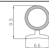
PERFIL: 1125
