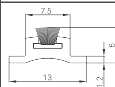
PERFIL: 5063
