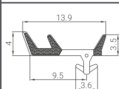
PERFIL: 2006
