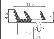
PERFIL: 2013
