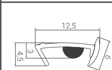
PERFIL: 1305
