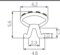
PERFIL: 1515
