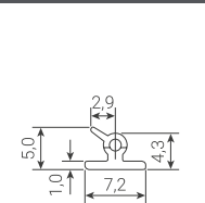
PERFIL: 5060
