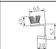
PERFIL: 1466
