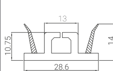
PERFIL: 5076
